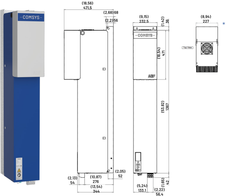
mm (inches) - PPM300v2B
